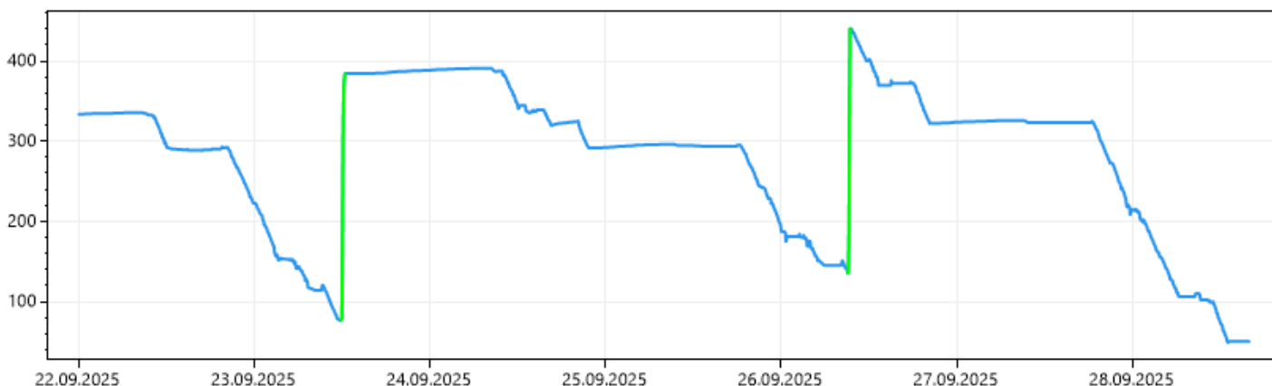
Уровень топлива от времени
